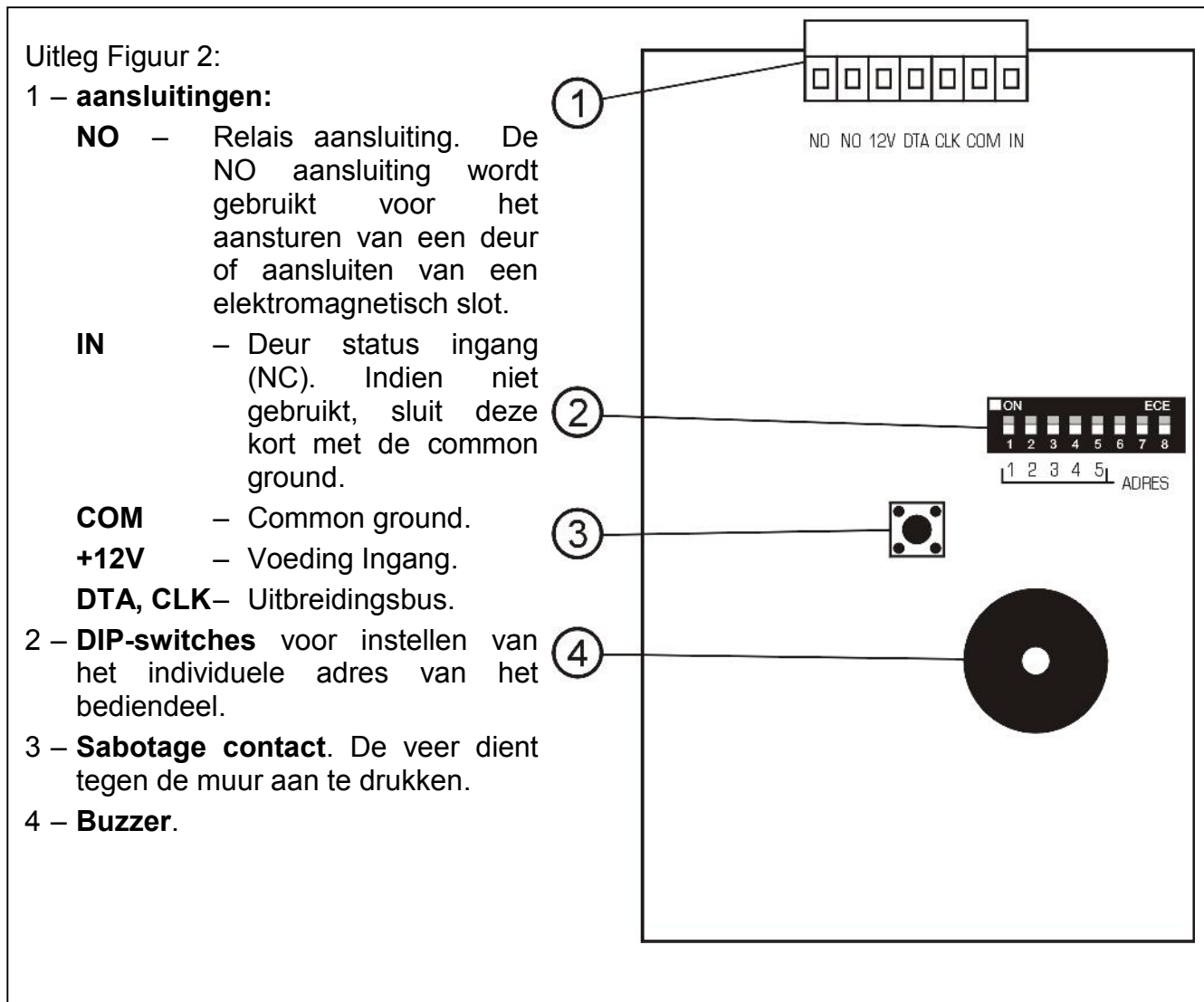
Figuur 2. Print overzicht van het bediendeel.
