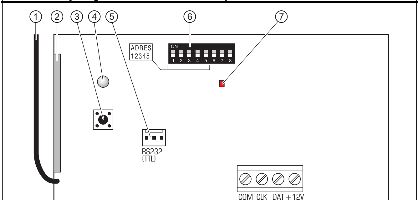
Fig. 1. Overzicht van de INT-RX uitbreiding module elektronica print.
