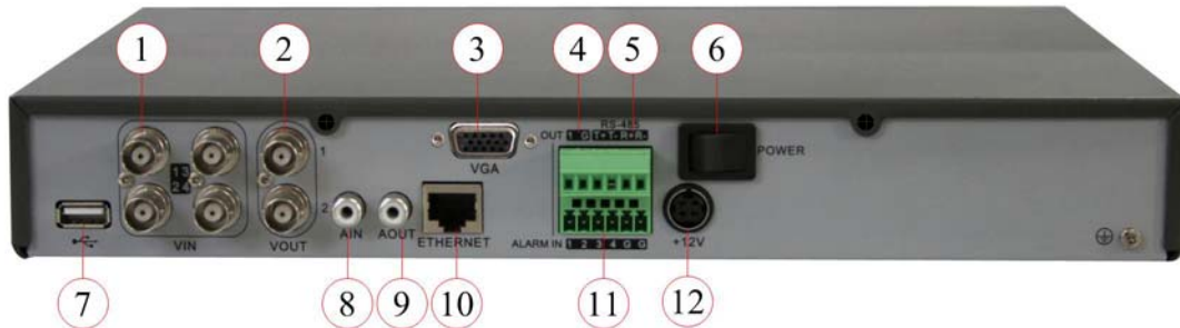
Fig. 2-1 DS-7204HVI-S Achterkant
